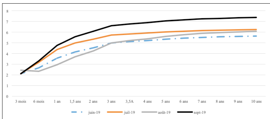
Graphique 11: Courbes de rendement des titres du Cameroun juin – septembre 2019
